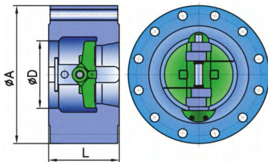
LUG TYPE
